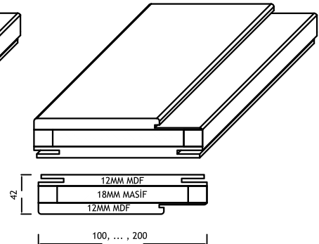
3 NOLU DÜZ KASA 3. no flat frame
