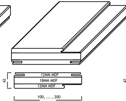
2 NOLU DÜZ KASA 2. no flat frame
